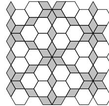
PATTERN 3 HEXAGON 01 - QTY 28 DIAMOND 01 - QTY 48
